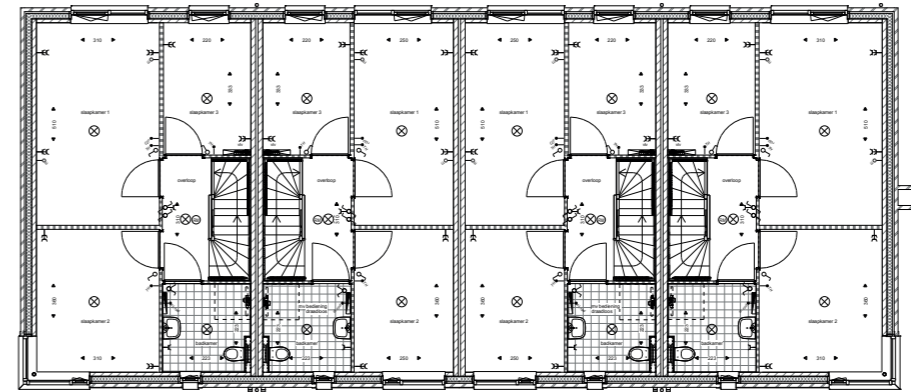
Eerste verdieping bouwnr 51 bouwnr 50 bouwnr 49 bouwnr 48
