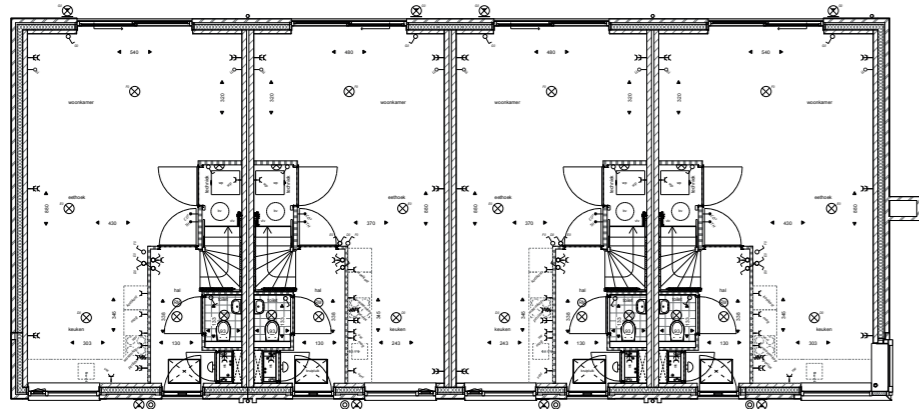
Begane grond bouwnr 51 bouwnr 50 bouwnr 49 bouwnr 48
