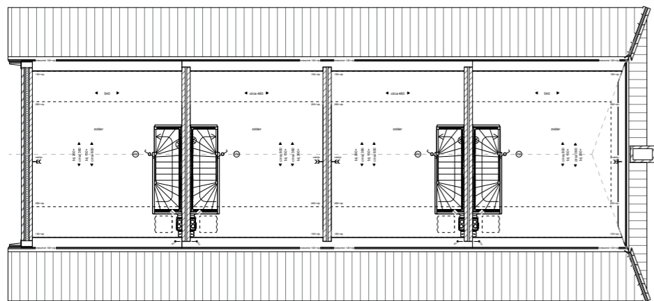
Tweede verdieping bouwnr 51 bouwnr 50 bouwnr 49 bouwnr 48
